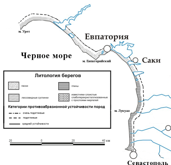
Р и с . 1 . Литологическое строение и противоабразионная устойчивость берегов Западного Крыма (показаны дочетвертичные породы и современные отложения крупных морских аккумулятивных форм).
