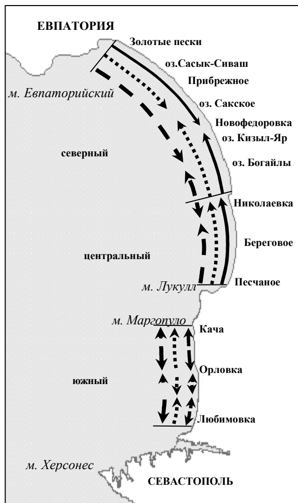
Р и с . 1 . Направление движения наносов: средне-многолетнее (1979 – 2008 гг.) (—); для теплых (— · —) и холодных (···) сезонов.
